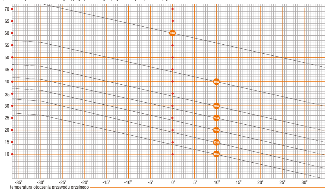
( W ) - moc jednostkowa samoregulującego przewodu grzewczego w danej temperaturze jego otoczenia
