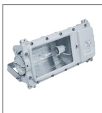
II 2G Ex de IIB T4-T3; II 2D Ex tD A21 T145°C-210°C; IP 66; HST/HIT; Kl. Ochr. I
